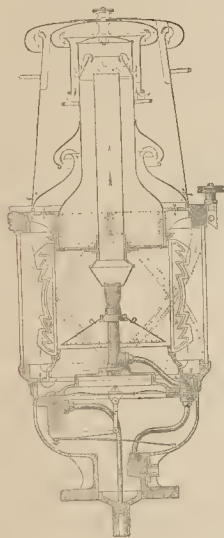
Fig. 5. Linterna de una boya luminosa; \frac{1}{8} de su verdadero tamaño
